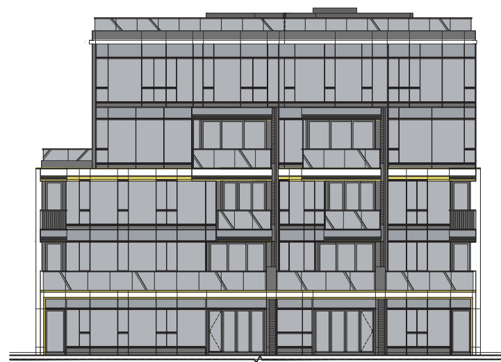
Elevation 1 立面圖1
