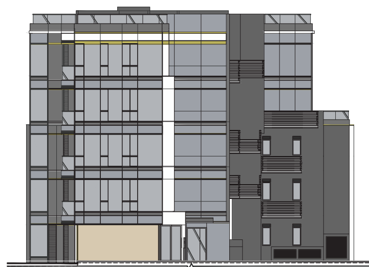
Elevation 3 立面圖3
